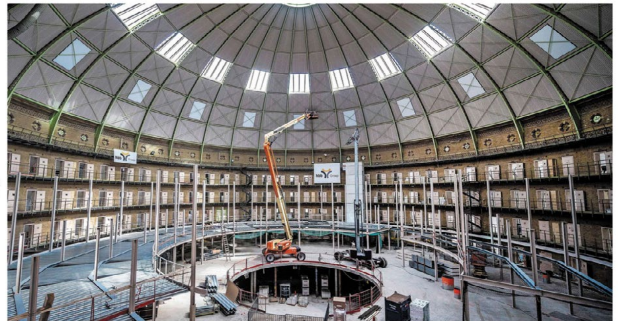
Er wordt hard gewerkt in de Koepel. Op de stalen constructie worden de kleine collegiazalen gebouwd.
